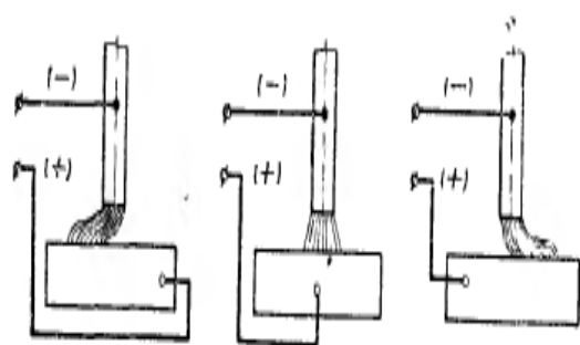
Рисунок 4. Влияние места подвода тока на отклонение дуги. Рисунок 5. Влияние ферромагнитных масс на отклонение дуги.
