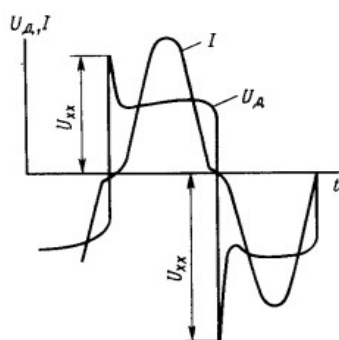
Рисунок 1. Исследование ионизирующего действия на дугу материалов покрытия электродов разных марок и флюсов Контрольные вопросы
