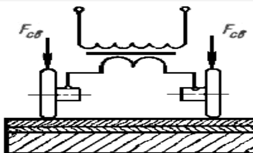
Рис.2. Односторонняя контактная шовная сварка
