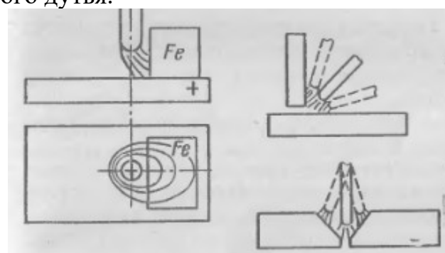
Рисунок 4. Влияние места подвода тока на отклонение дуги. Рисунок 5. Влияние ферромагнитных масс на отклонение дуги.
