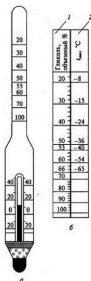
Рис. 1. Гидрометр (а) для определения температуры застывания и содержания этиленгликоля в антифризах и его шкала (б): 1 — шкала «Глицоль, объемный %»; 2 — шкала температуры замерзания t_{зам}
