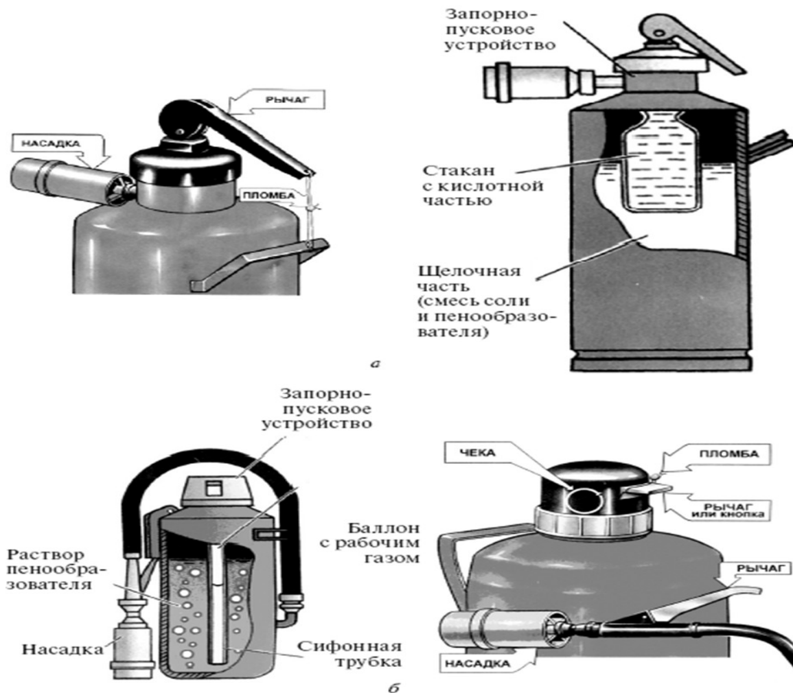
Рис 1. Ручные огнетушители: а – химический пенный огнетушитель ОХП-10; б – воздушно-пенный огнетушитель ОВП-10
